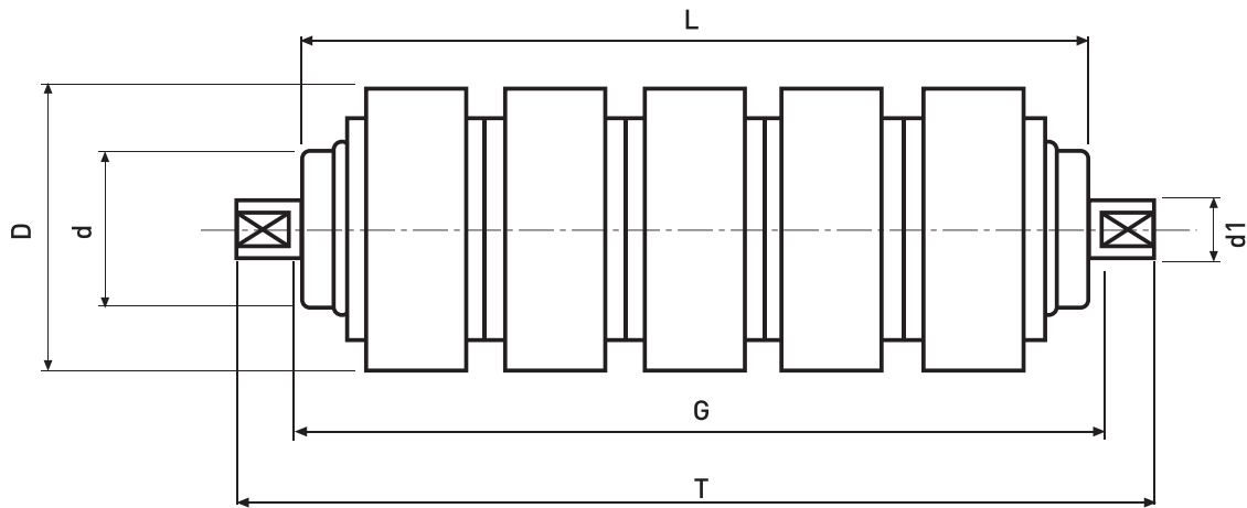
Rodillo amortiguador.
