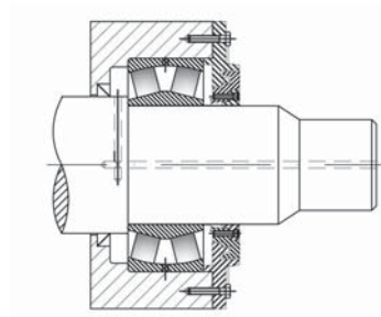
b- Rodamientos
