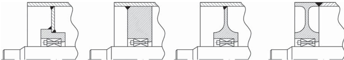
1-Cubo con disco soldado
