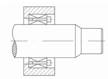
a- Anillos de presión o unidades cónicas
